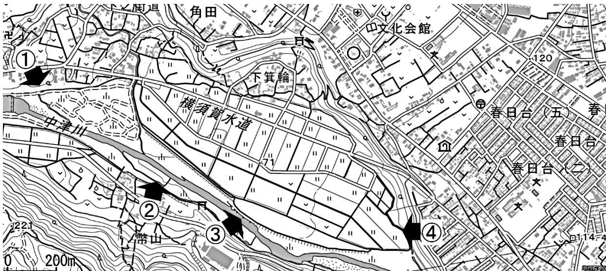
神奈川県愛甲郡愛川町域の地形図（画像取得 2023 年 地理院地図を改変）
